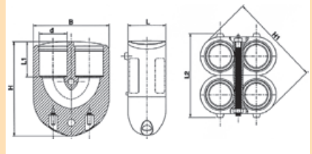
Abmessungen ENREGIS/Sondenkopf
